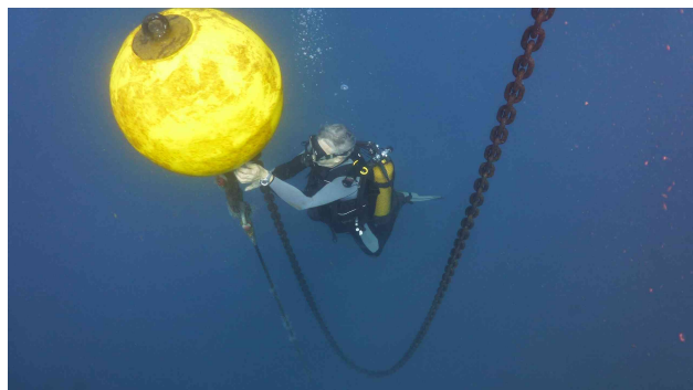
Figure 21 : Manillage d'un coffre sur le flotteur subsurface
