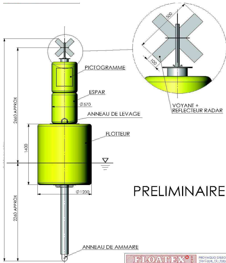
Figure 10 : Bouée de « marque spéciale »
