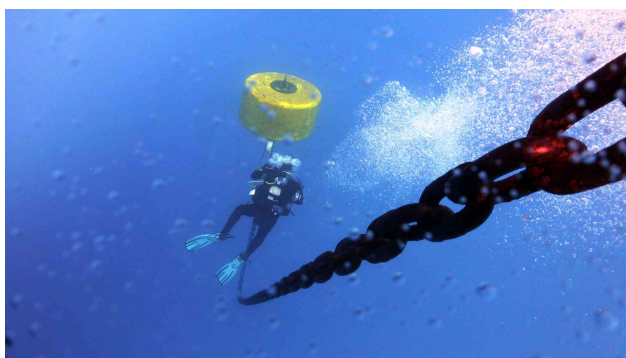
Figure 23 : Manillage d'une bouée sur le flotteur subsurface
